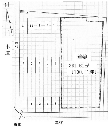
T N店舗【木太町】配置図 ※図面と異なる場合は現況優先とします。
